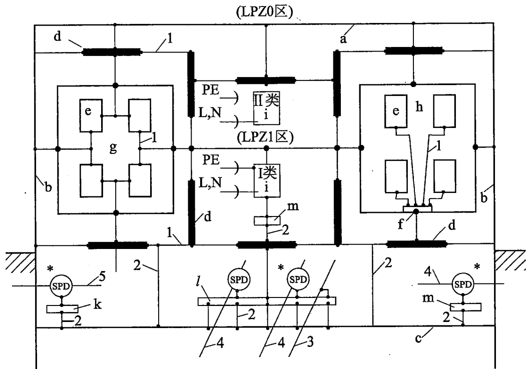
图 6.3.3 接地、等电位连接和接地系统的构成
