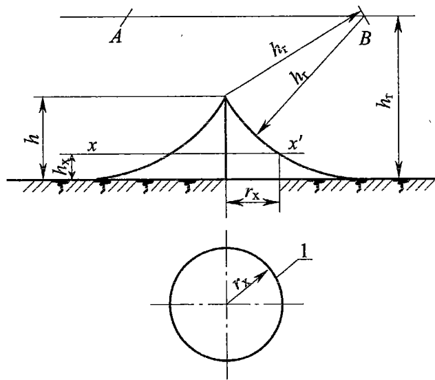
图 D.0.1 单支接闪器的保护范围
