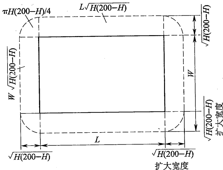
图 A.0.3 建筑物的等效面积
