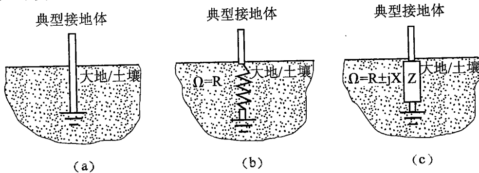
图 3 典型接地体的三种表示
