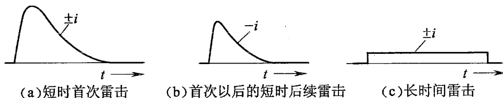
图 F.0.1-1 闪电中可能出现的三种雷击
