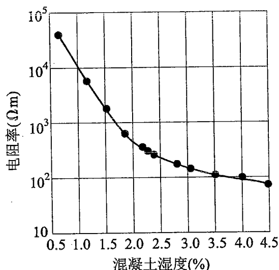
图 12 混凝土湿度对其电阻率的影响
