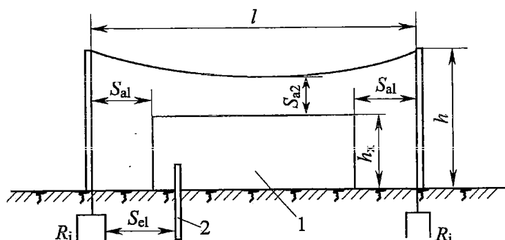
图 4.2.1 防雷装置至被保护物的间隔距离
