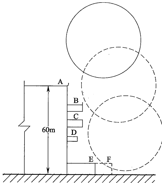
图 14 剖面示意
